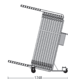
Uskladňovací vozík 6398-000 (příklad při délce stolu 1600)
